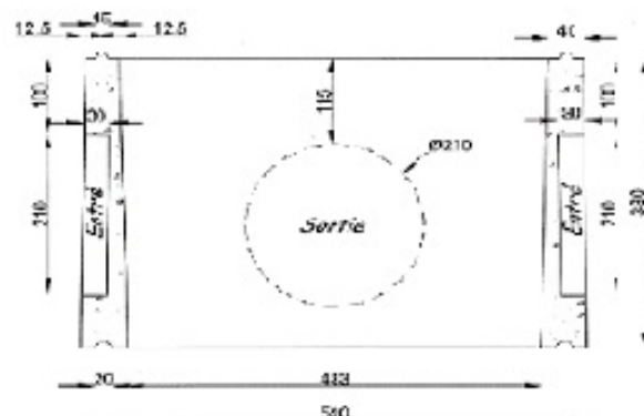
REHAUSSE 500X500
