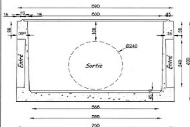
REGARD 600X600
