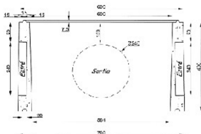
REHAUSSE 600X600
